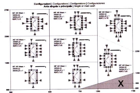
Tipi di configurazioni degli accessori antieffrazione a seconda delle dimensioni per anta singola e doppia
